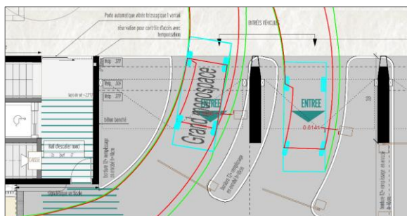
Test des rayons de giration dans les chenaux d'accès du parking P1 sur la base des plans d'architectes APD – Source Sareco
